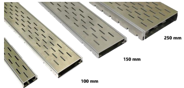
Abbildung 1: VOLFI Drainroste in Kombination mit optional erhältlichen VOLFI Kastenrinnen. Breite = Gesamtbreite der Kombination
