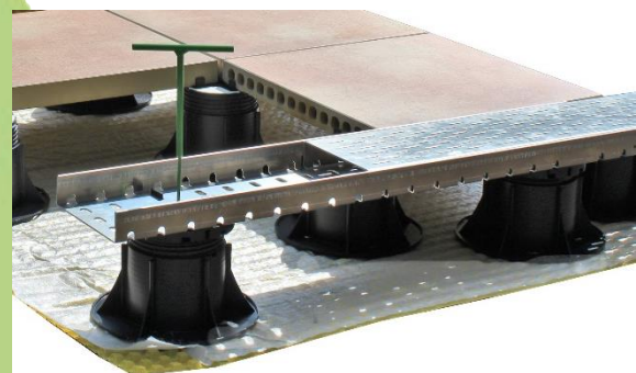
Abbildung 2: VOLFI Drainrost exemplarisch eingebaut in einen Plattenverbund. Entsprechende Kastenrinne und Volfiteller VT-B 4/10 erforderlich. Stelzen = SV-403; auf Drainmatte DRM
