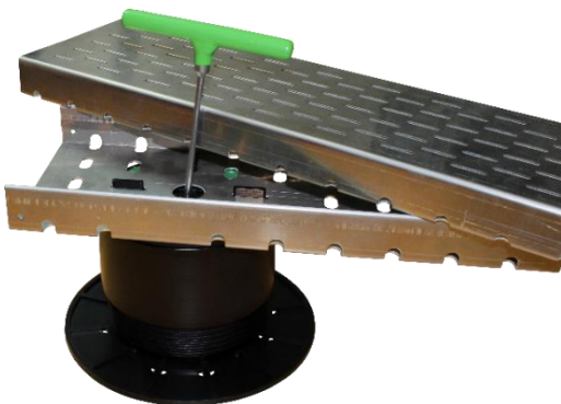
Abbildung 8: Kastenrinne aufgestellt auf Stelzlager TL-V mit eingesetztem VOLFI Stellschlüssel zur nachträglichen Feinjustierung.
