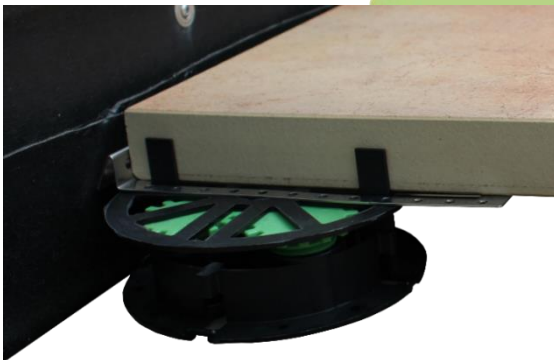
Abbildung 2: Anwendungsbsp. Wandabstandhalter eingelegt in Stelzlager ZR-V35
